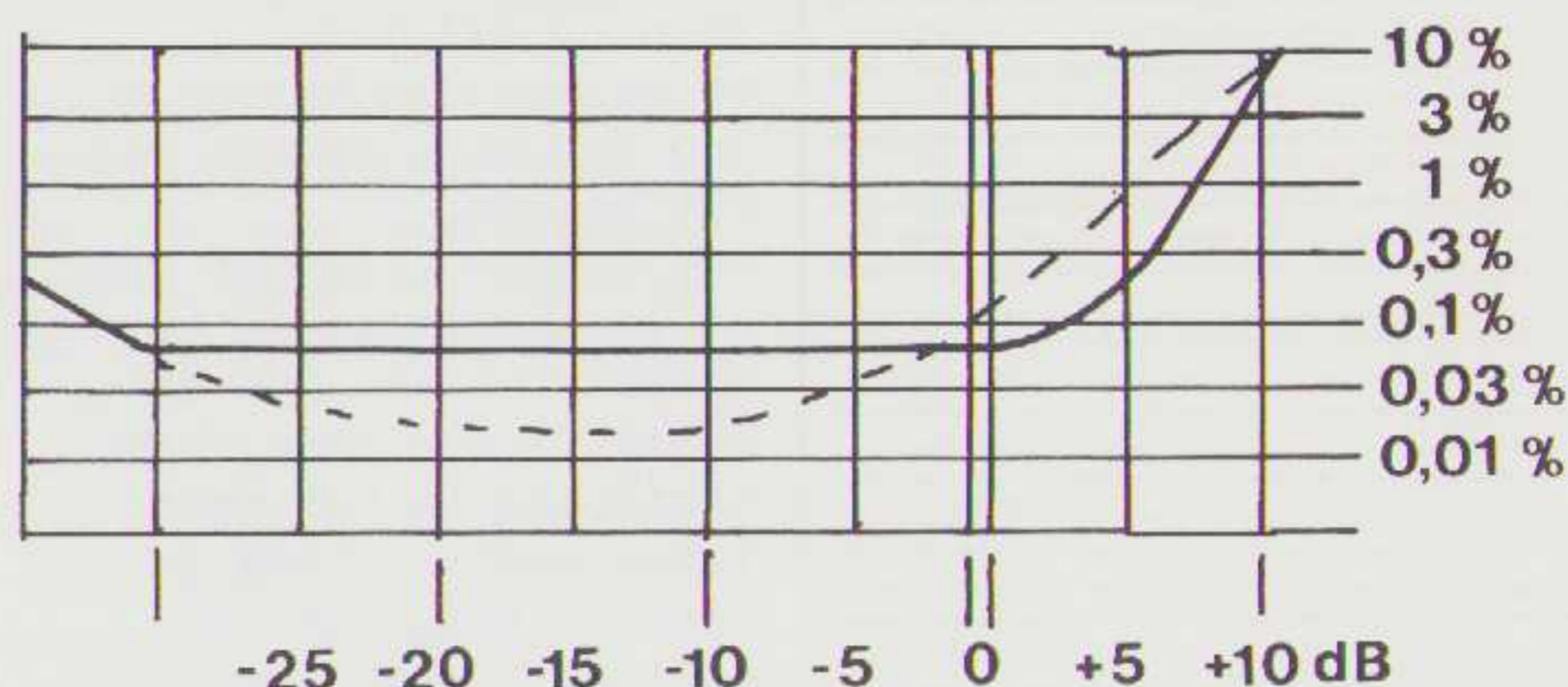
VERVORMINGSKARAKTERISTIEK
